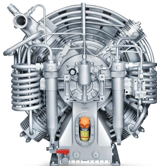
IK 150 Compressor Block
